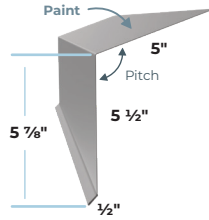
RPLE RP Long Eave
