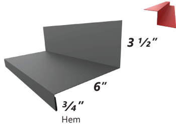
SL6SW SL Sidewall
