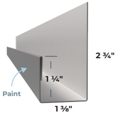
RPFJ1 RP 1-3/8" F&J
