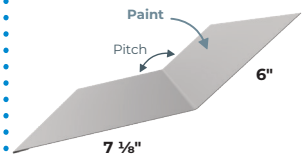
RPLG RP Lower Gambrel
