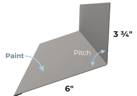
RPEW RP Endwall
