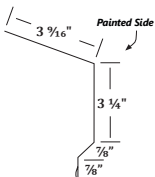
EF 5 Eave Facsia
