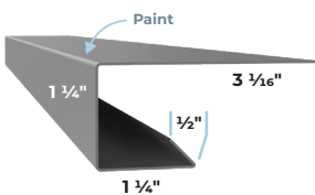
RPJT RP Jamb Trim
