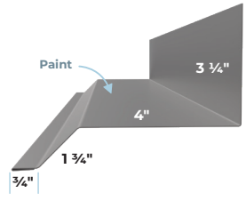
RPEW RP Endwall
