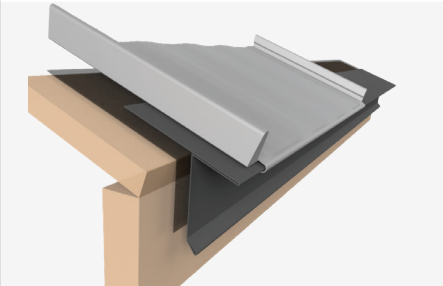
SL6SW SL Sidewall
