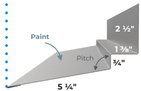
RPLG RP Lower Gambrel
