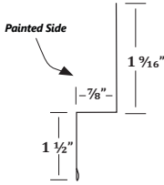
DA 1-1/2" Double Angle
