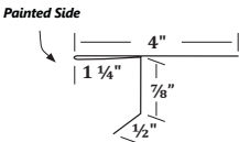
DE114 1-1/4 Drip Edge
