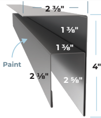
RPFJ1 RP 1-3/8" F&J
