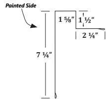
SDJ Sliding Door Jamb
