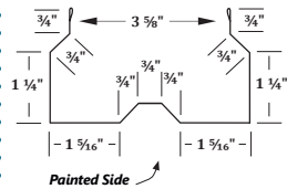
YL615 YL615 Post Wrap
