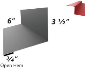
SL6EW SL Endwall
