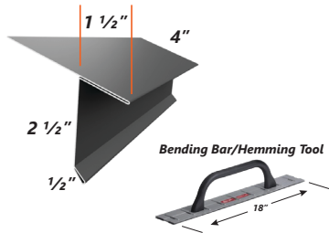
SL6DE SL Drip Edge
