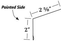
GA Gutter Apron
