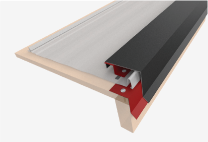
SL6EW SL Endwall
