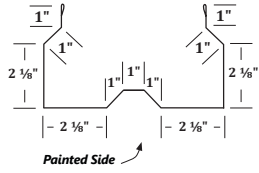
YL240 YL240 Post Wrap
