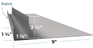
RPODJ RP Overhead Door Jamb
