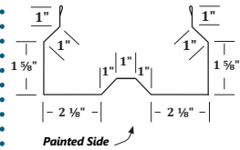
YL550 YL550 Post Wrap
